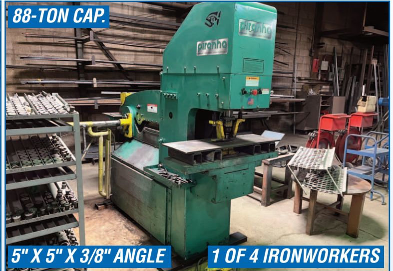
PIRANHA PII88 IRONWORKER
