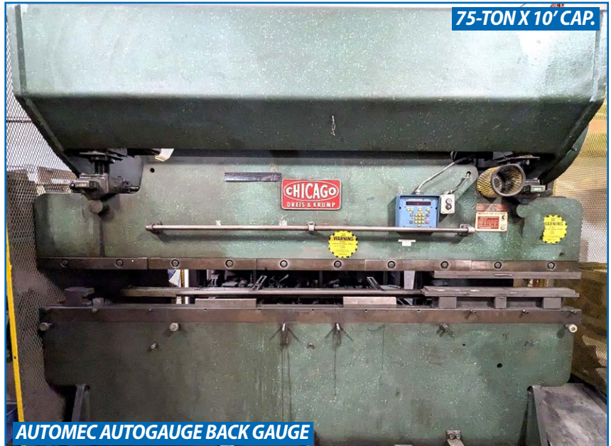
CHICAGO / DREIS & KRUMP 810-C PRESS BRAKE
