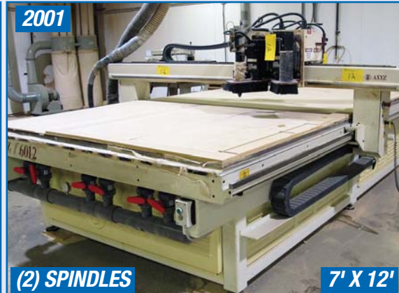
AXYZ 6012 CNC ROUTER
